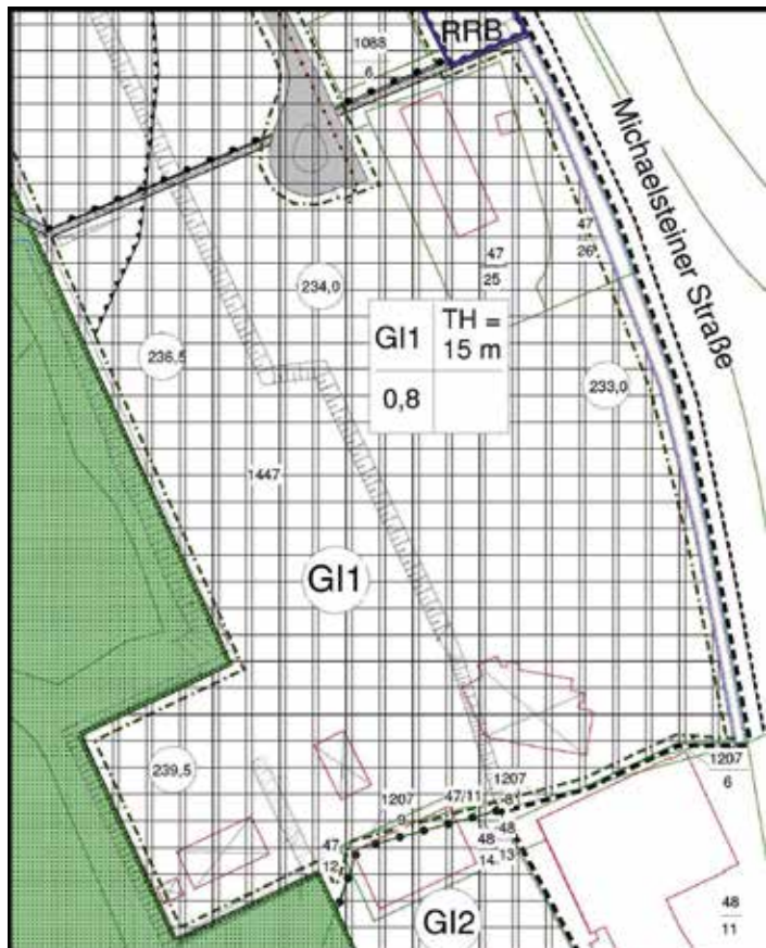
Übersichtsplan mit dem Geltungsbereich der 1. Änderung des B-Planes "Gewerbegebiet Oesig", Blankenburg (Harz) Gemarkung Blankenburg, Flur 2 unmaßstäblich
